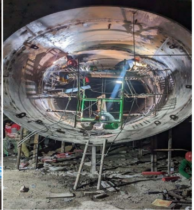
लोअर क्षैतिज पीएस का द्विभाजन - 3.9 मी व्यास, एमआईवी का अप /स्ट्रीम
