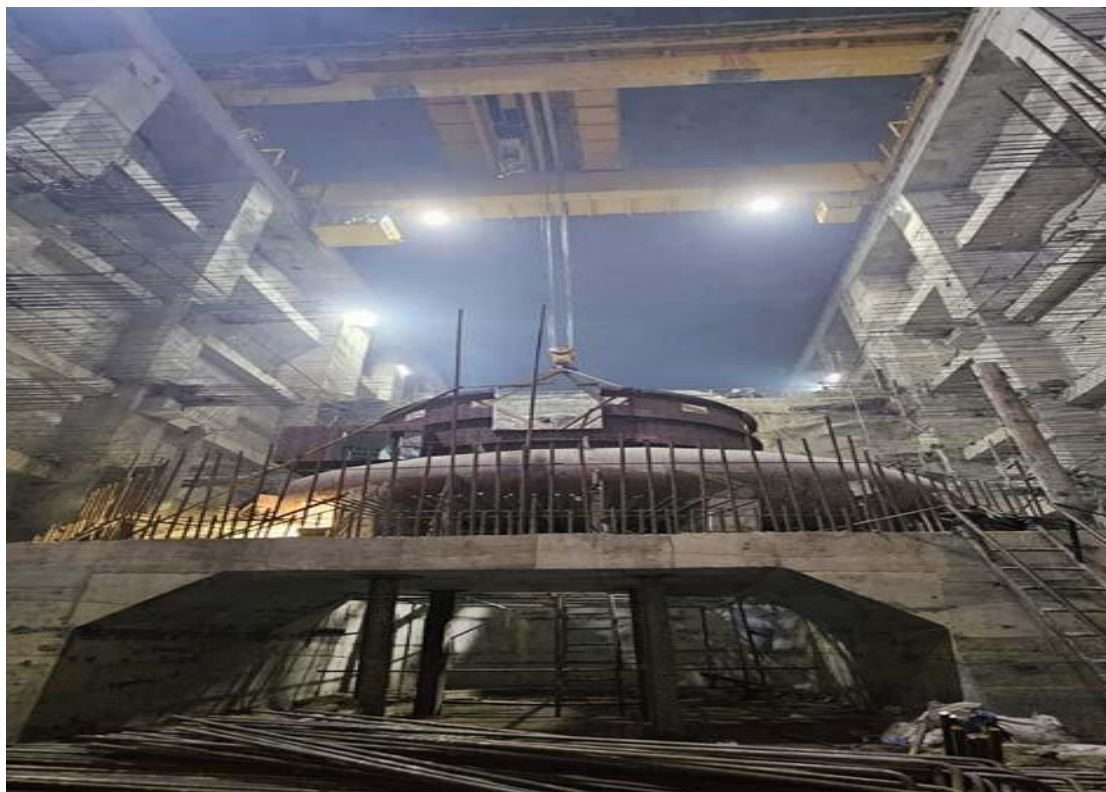
यूनिट-1 पिट लाइनर
